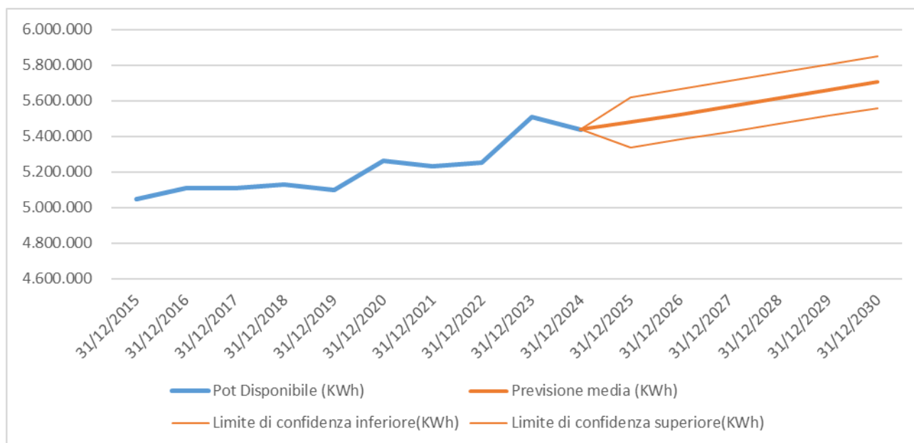
Grafico 8: Previsione di crescita della Potenza Disponibile agli utenti BT e MT al 31/12/anno-n, da serie storica e limite di confidenza 95%
